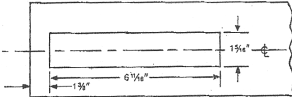
Aluminum frame door header
